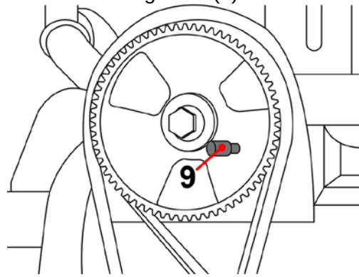
Pasador de bloqueo del árbol de levas / cigüeñal (9)
