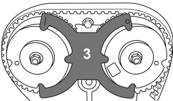
Herramienta de ajuste VCT (3)
