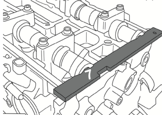
Outil de réglage d'arbre à cames (7)
