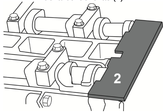
Herramienta de sincronización del árbol de levas (2)
