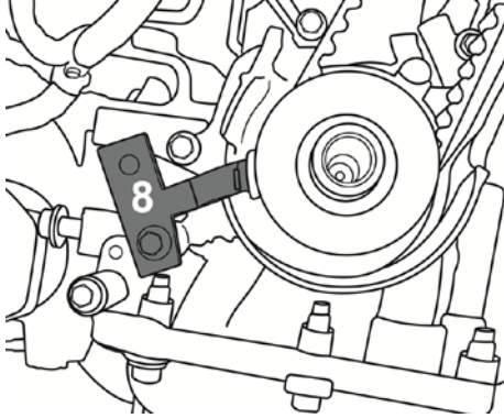
Riemenscheiben-Einstellwerkzeug (8)
