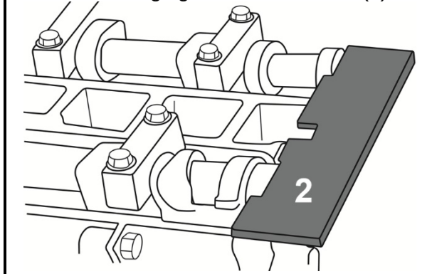
Outil de réglage d'arbre à cames (2)
