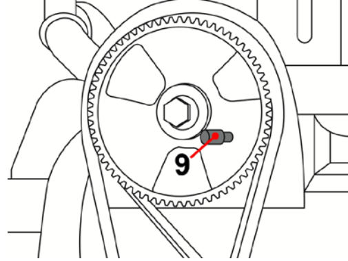
Nocken-/Kurbelwellen-Einstellstift (9)
