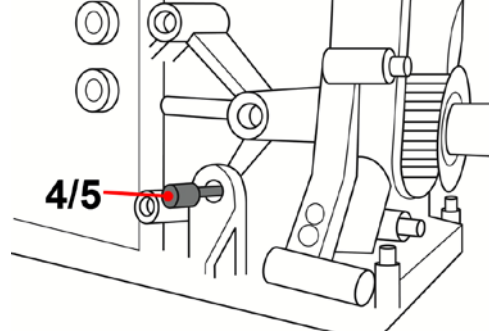
Pasador de sincronización del cigüeñal (4/5)
