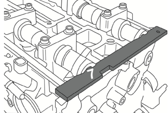
Nockenwellen-Einstellwerkzeug (7)
