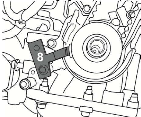
Outil de réglage de poulie (8)
