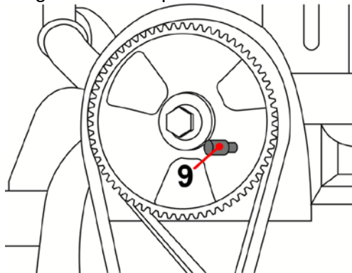
Blocage de vilebrequin/ l'arbre à cames (9)
