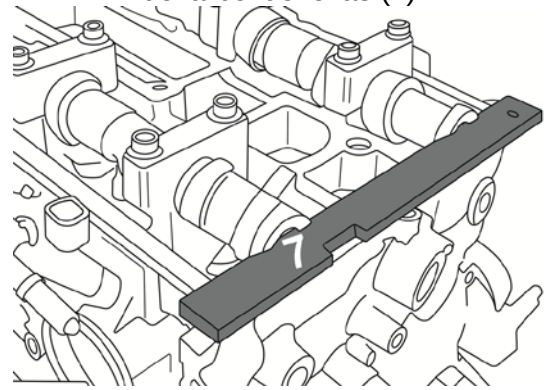
Herramienta de sincronización del árbol de levas (7)
