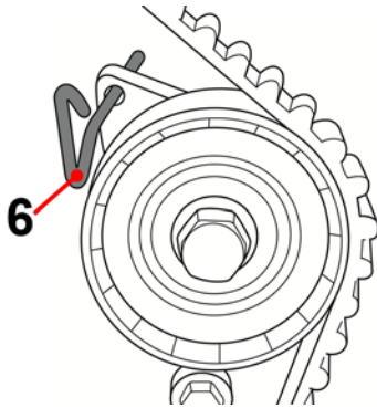
Spannrollen-Arretierstift (6)
