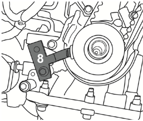
Herramienta de ajuste de poleas (8)
